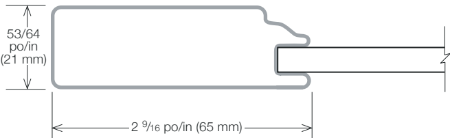
PLAT / FLAT
