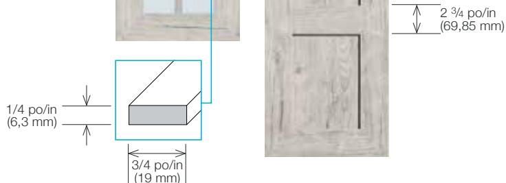
PLAT / FLAT
