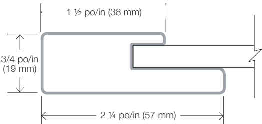
PLAT / FLAT
