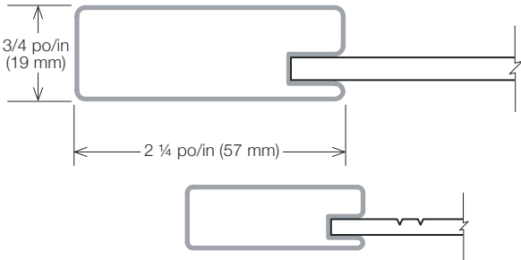
PLAT / FLAT
