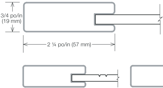
PLAT / FLAT
