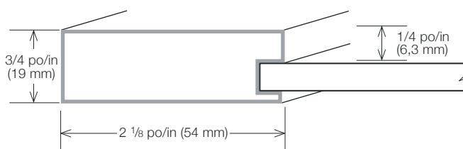
PLAT / FLAT
