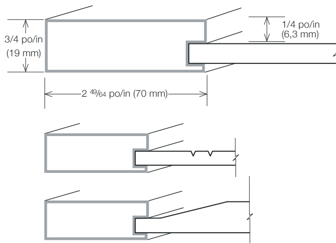
PLAT / FLAT
